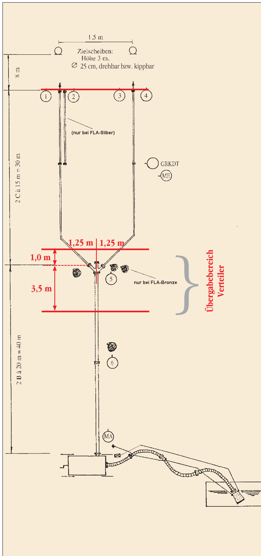
Skizze 2: Endaufstellung nach Beendigung des Löschangriffes.
